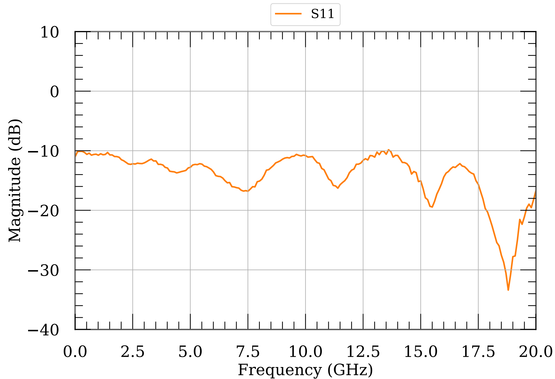
LNA S-params module039
